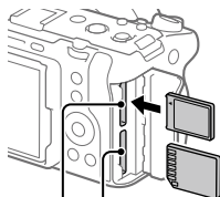
Слот 1 Слот 2
