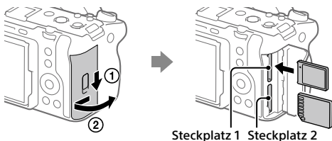
Steckplatz 1 Steckplatz 2
